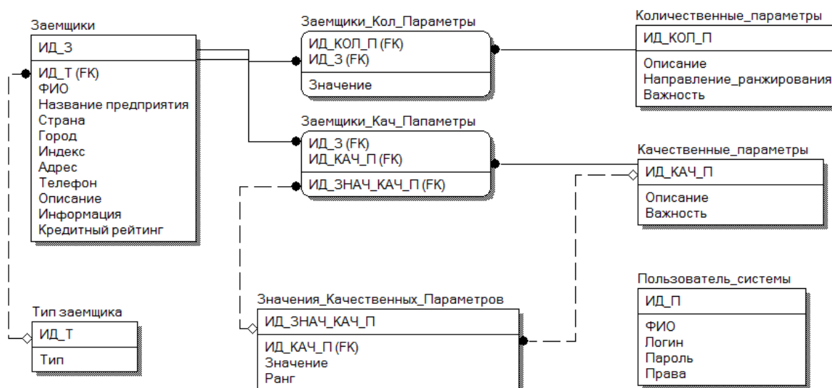
Рисунок 2. Даталогическая модель
