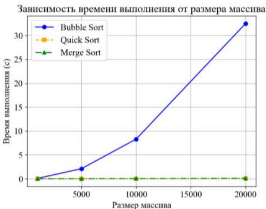
Рисунок 1. График зависимости времени от размера массива
