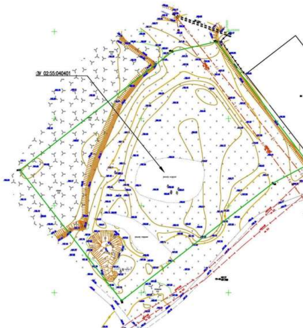
Рисунок 3. Общий вид топографического плана
