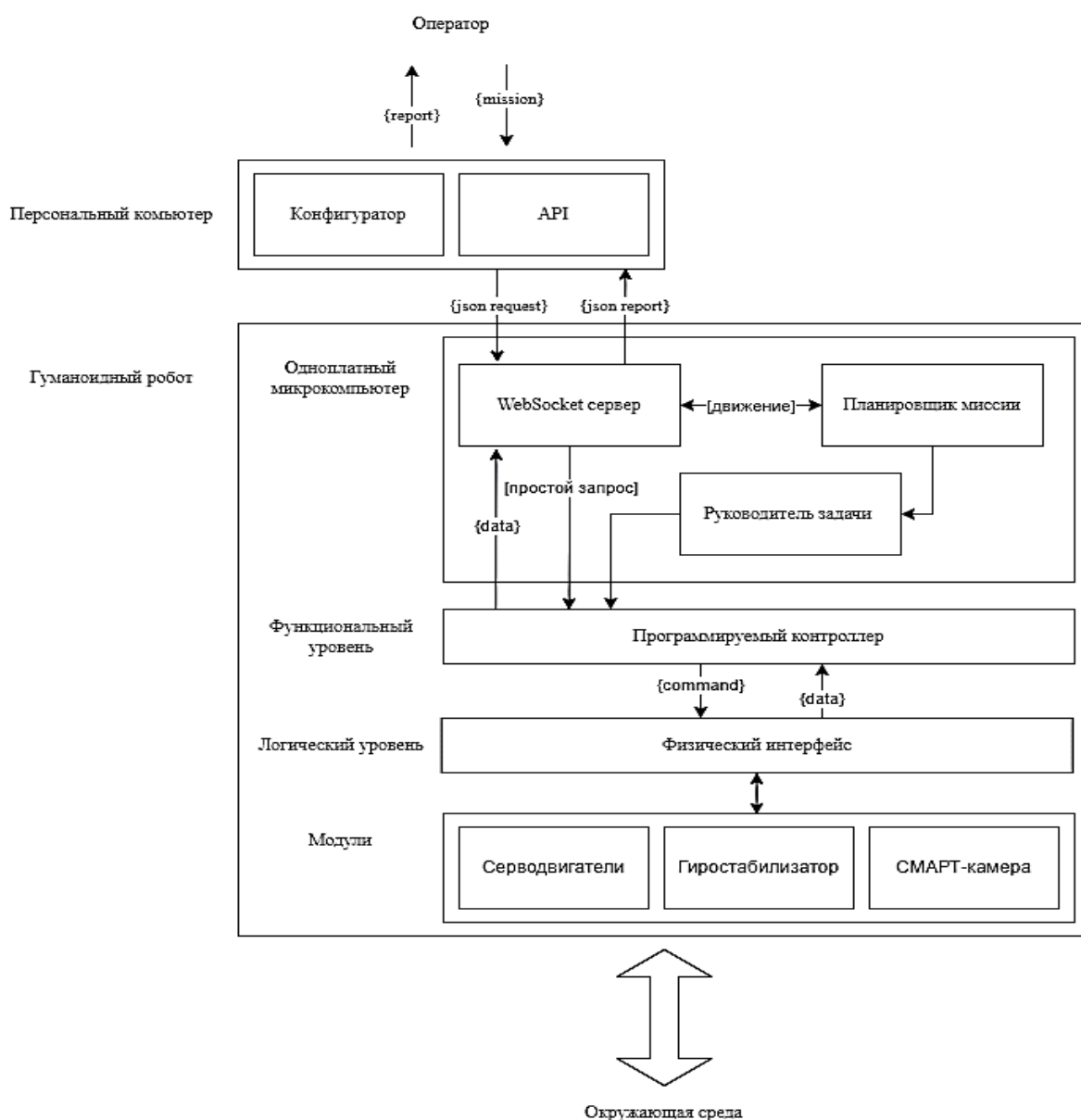
Рисунок 2. Схема взаимодействия гуманоидного робота
