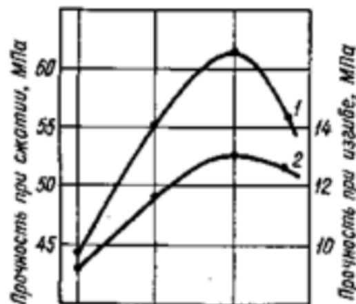
Рисунок 4. Влияние содержания ПВА на прочность цементного камня после 28 сут. твердения 1 — при сжатии; 2 — при изгибе
