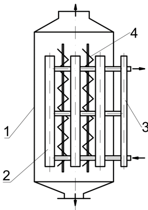
Рисунок 1. Охладитель зерна
