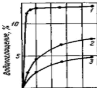
Рисунок 5. Зависимость водопоглощения от времени водного твердения 1 — цементного камня; 2 — модифицированного латексом, П/Ц = 0,05; 3 — то же, П/Ц = 0,2
