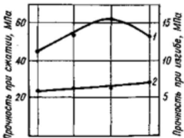
Рисунок 3. Влияние содержания поливинилового спирта на прочность цементного камня после 28 сут. твердения 1 — при сжатии; 2 — при изгибе
