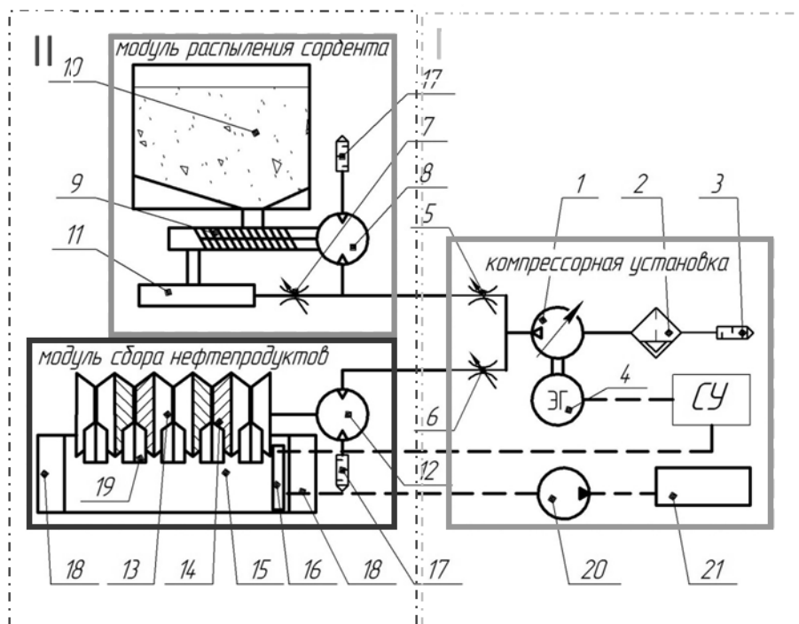
Рисунок 1. Технико-функциональная схема работы комбинированного устройства, где 1 - регулируемый компрессор, 2 - фильтр, 3, 17 - шумогаситель, 4 - электрогенератор, 5, 6, 7 - дроссель, 8, 12 - пневмомотор, 9 - шнек, 10 - бункер сорбентом, 11 - сопло, 13, 14 - секции нефтесборщика, 15 - бак для сбора, 16 - уровнемер, 18 - воздушные камеры, 19 - приемные лотки, 20 - насос откачки, 21 - бак хранения нефтешлама; I - модуль, устанавливаемый на суше/ судне; II - модули, устанавливаемые в акватории водоема
