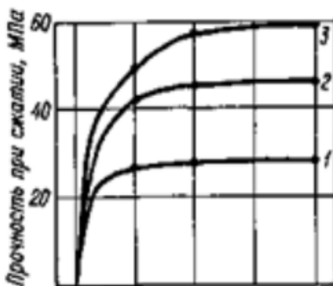
Рисунок 2. Влияние продолжительности твердения на прочность при сжатии модифицированного латексом цементного камня 1 - без добавки; 2 - П/Ц = 0,15; 3 - П/Ц = 0,2.
