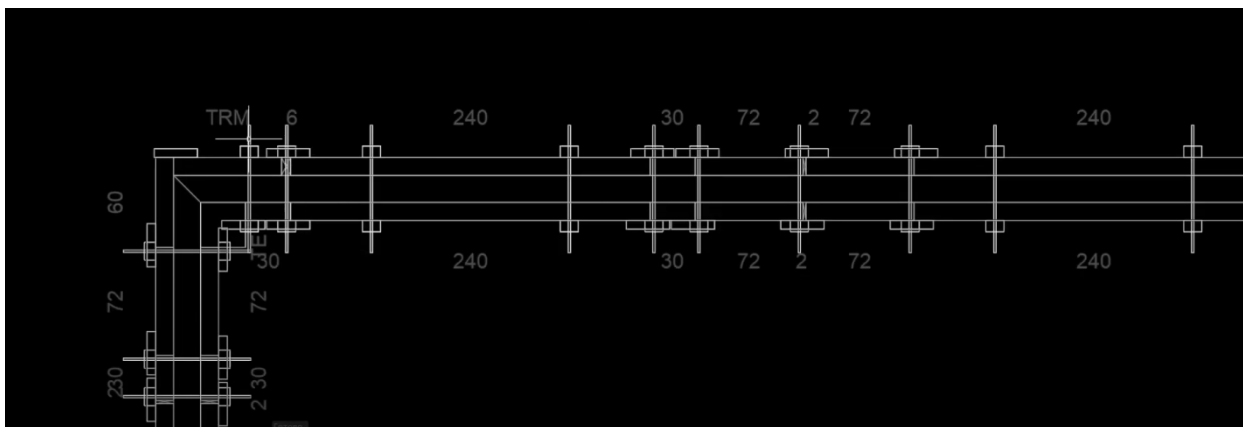
Рисунок 7. Разложенная опалубка и ее элементы
