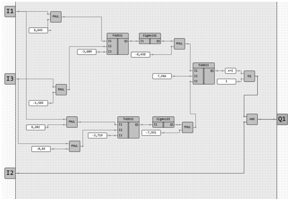
Рисунок 2. Программная реализация нейросети в OWENLogic
