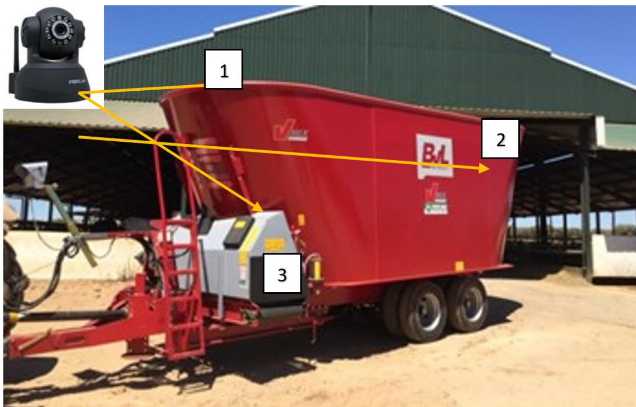
Рисунок 1. Возможный вариант установления видео устройств на смесителе-кормораздатчике: 1, 2 – в корпусе бункера; 3 – на ленточном транспортере
