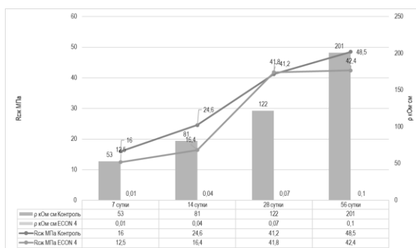
Рисунок 1. Результаты механических и электротехнических испытаний серии образцов контрольного и электропроводящего (ЕСОН 4) составов
