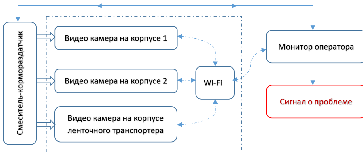
Рисунок 2. Принципиальная схема работы видео устройства при установке его на смесителе-кормораздатчике
