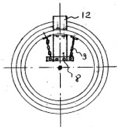
Рисунок 2. Дыхательный клапан в разрезе
