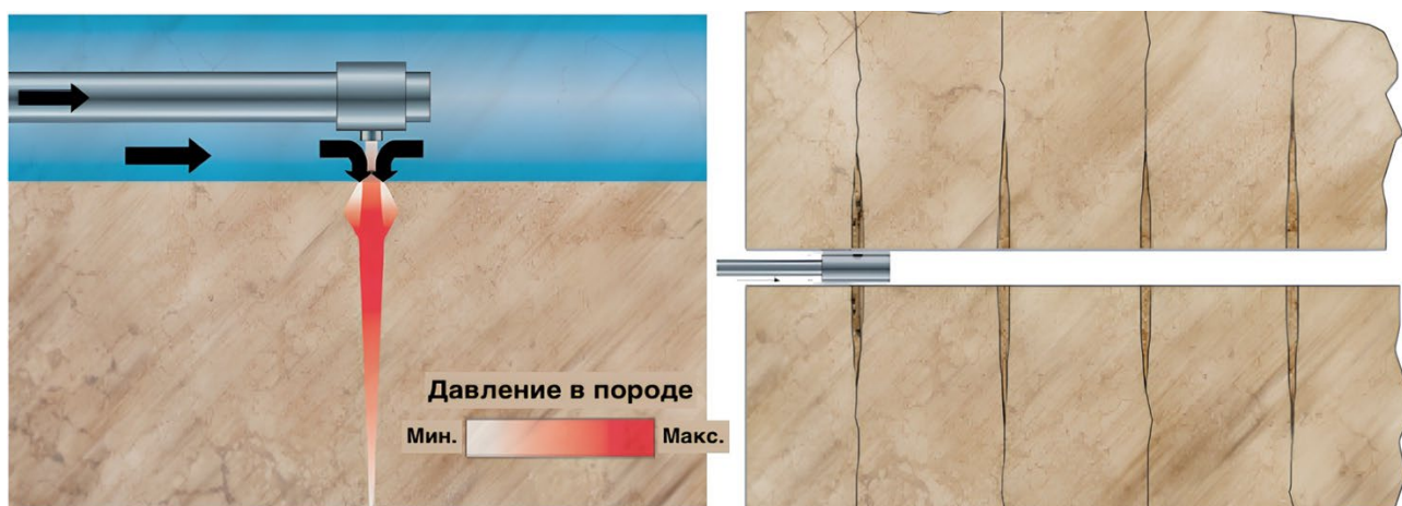
Рисунок 2. Схема эксплуатации инструментальной компоновки «Hydra-Jet™»
