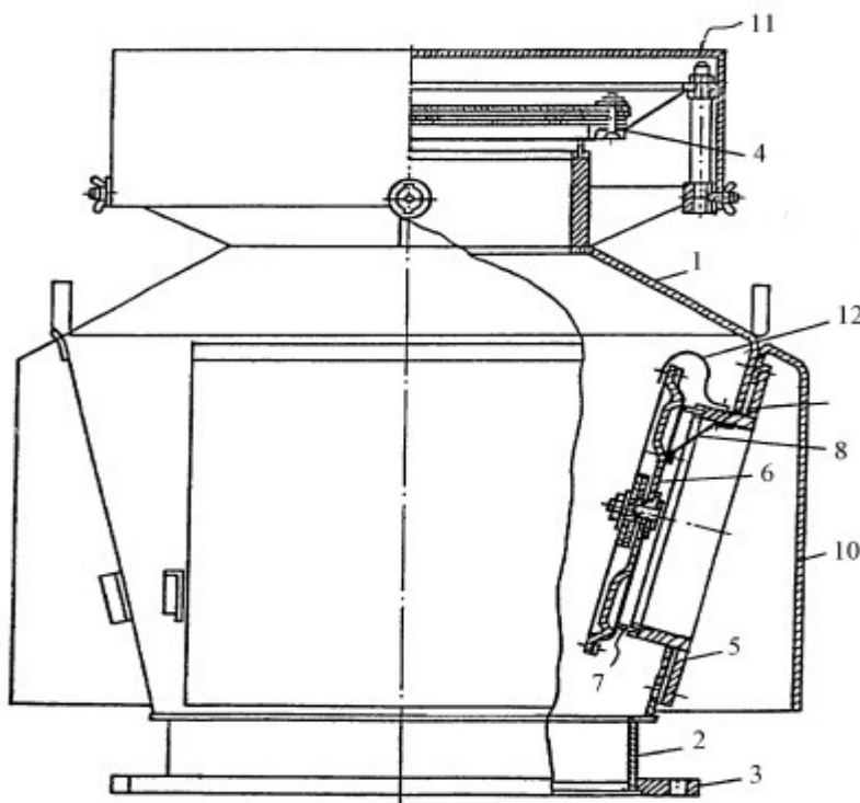
1- Корпус, 2- патрубок, 3- соединительный фланец, 4- затвор, 5- непромерзающий затвор, 6- тарель, 7 седло, 8- основная гибкая связь, 10- кожух, 11- крышка, 12- предохранительная гибкая связь
