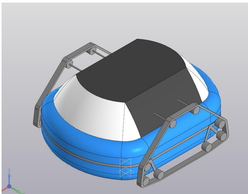
Рисунок 4. Трёхмерная модель подводного аппарата для очистки бортовых частей судов
