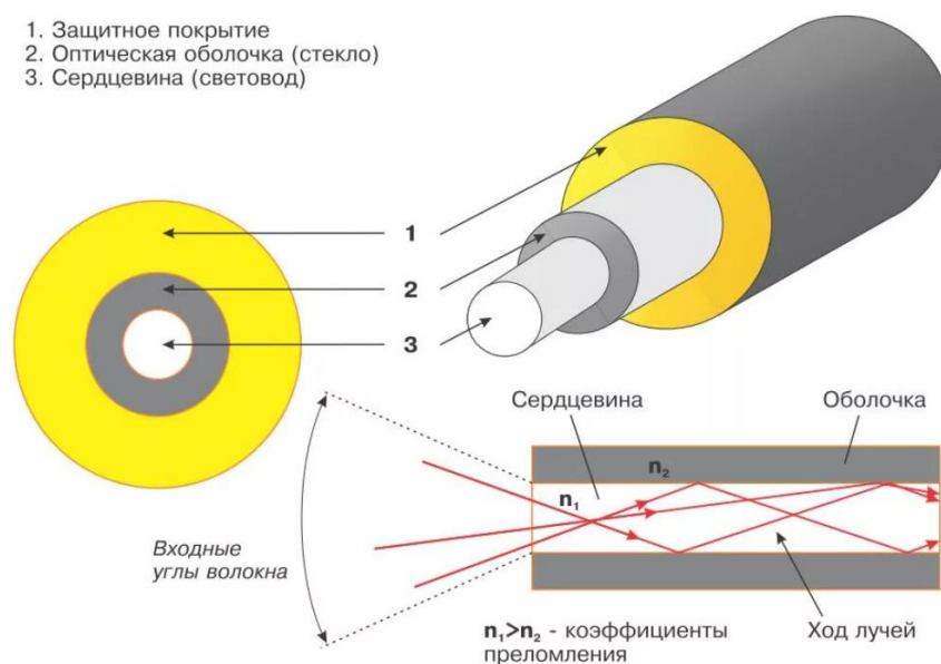
Рисунок 1. Структура оптоволокна
