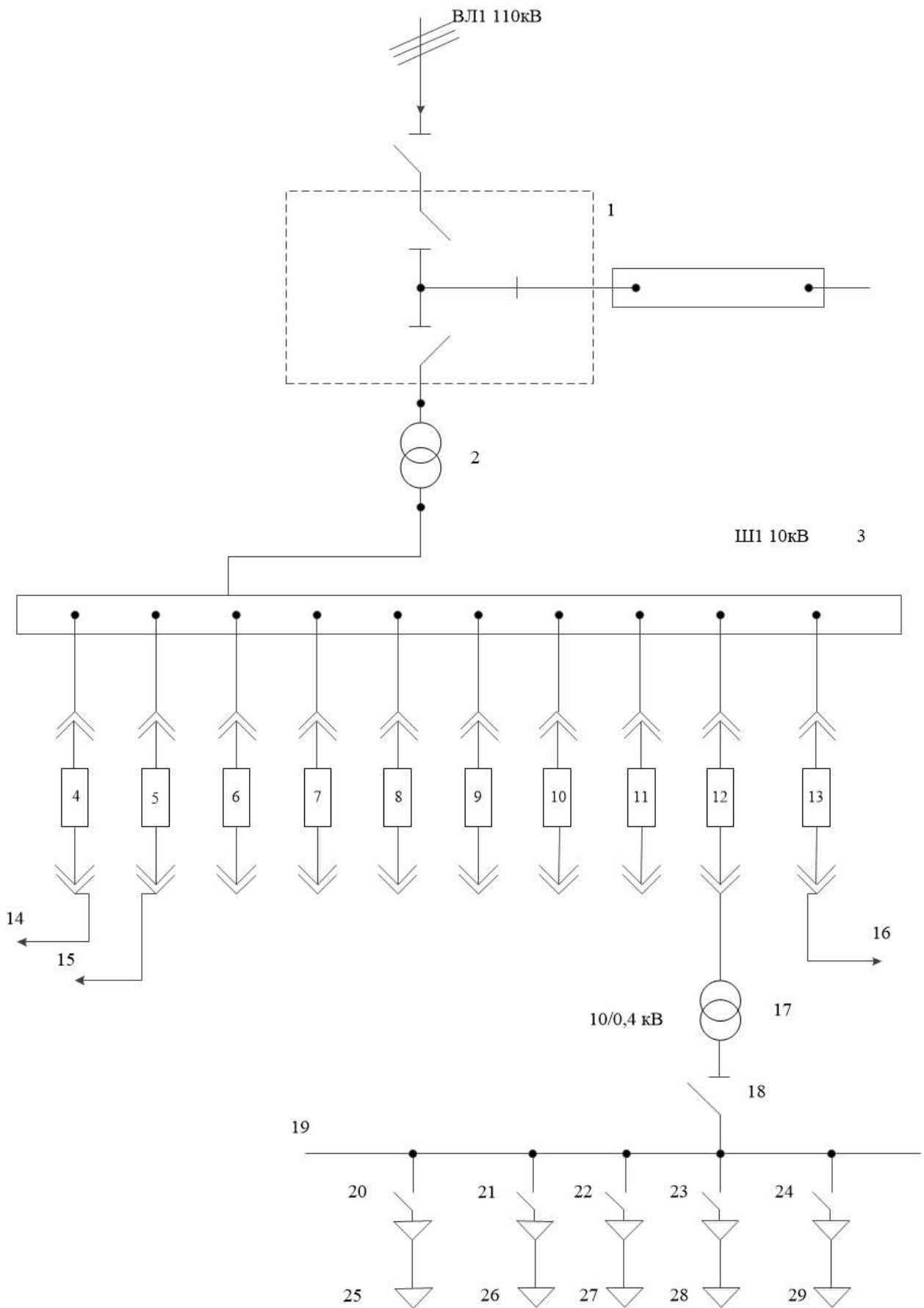
Рисунок 2. Структурная упрощенная схема ТП для одной ВЛ БГКМ
