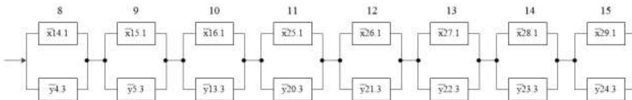
Рисунок 4. Схем минимальных сечений учитывающая отказ выключателей/разъединителей в срабатывании
