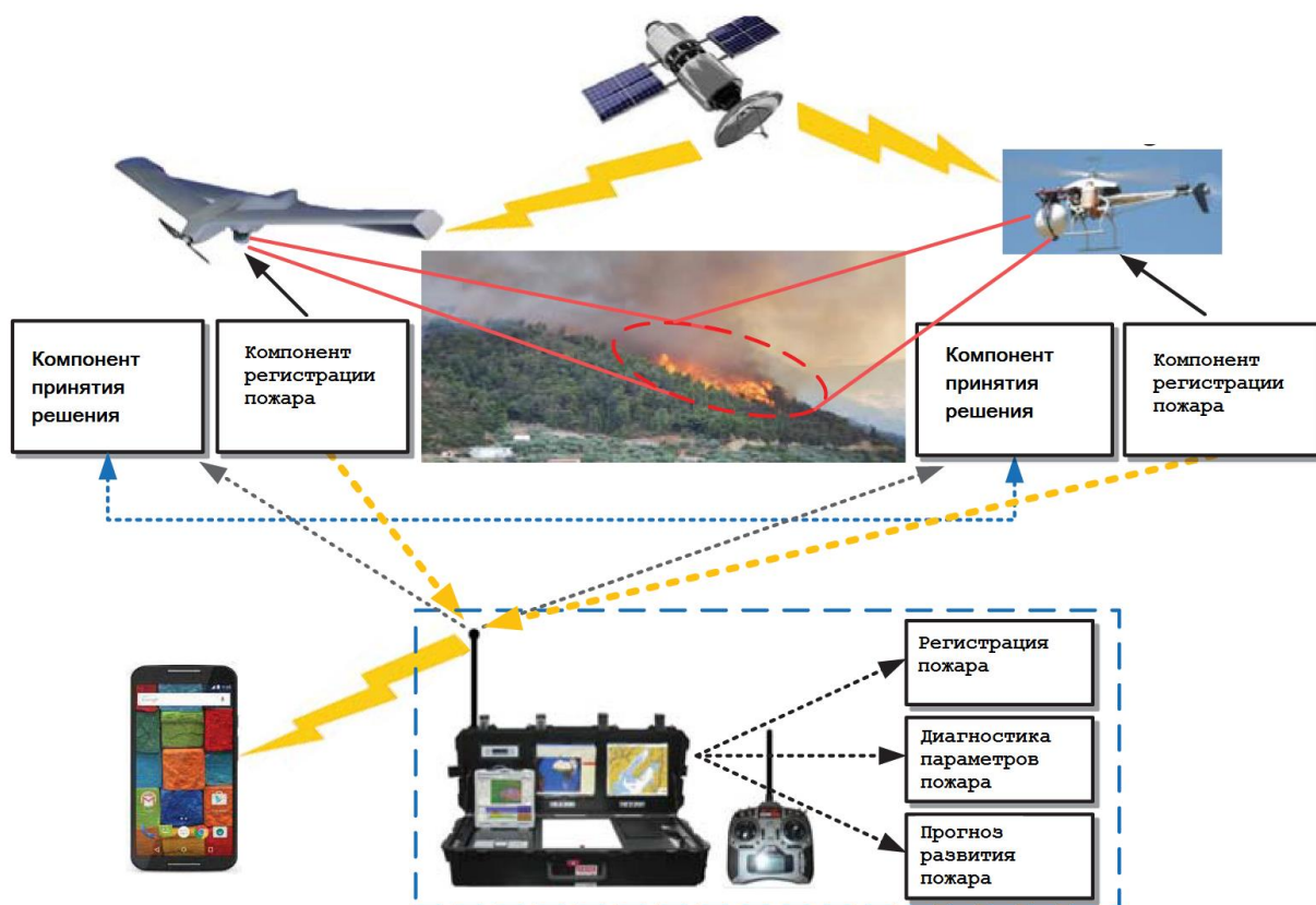
Рисунок 1. Основные компоненты общей системы наблюдения за лесными пожарами
