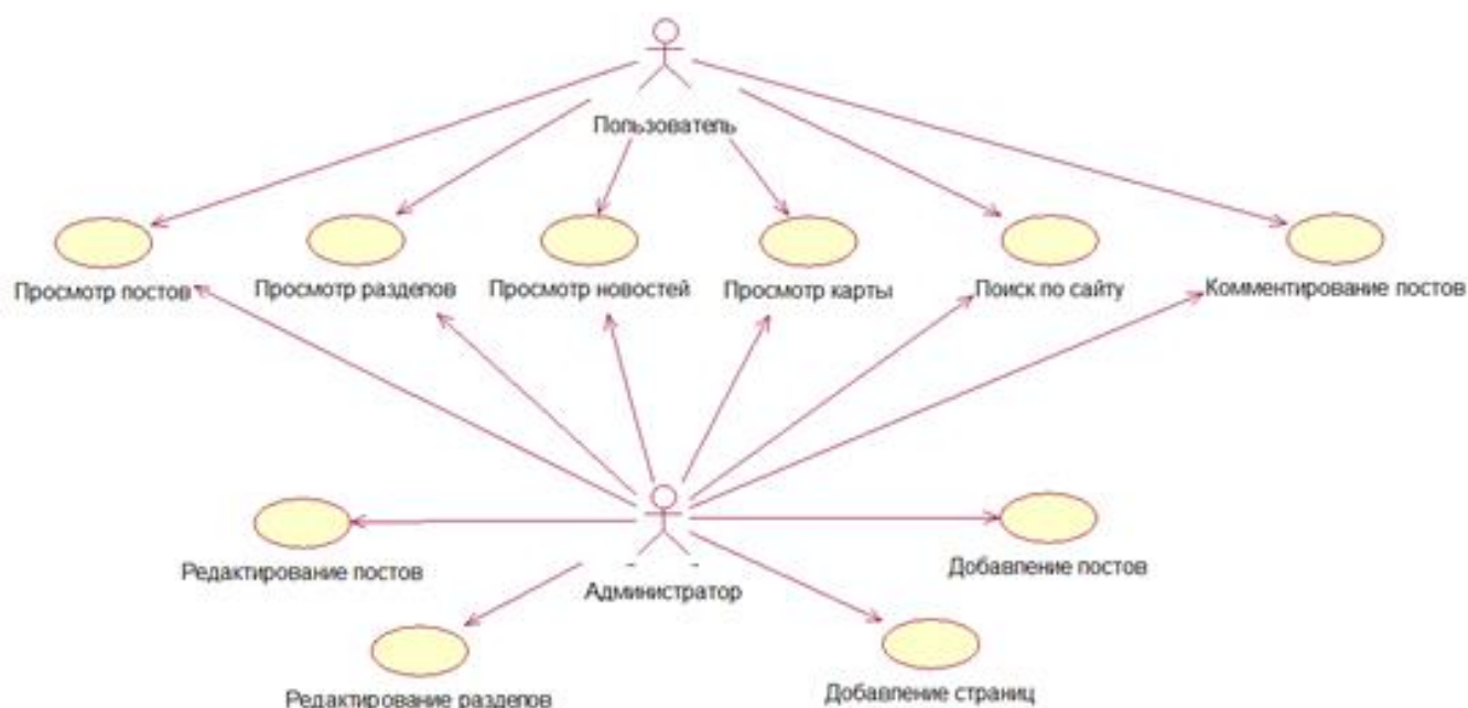
Рисунок 2 . Диаграмма вариантов использования
