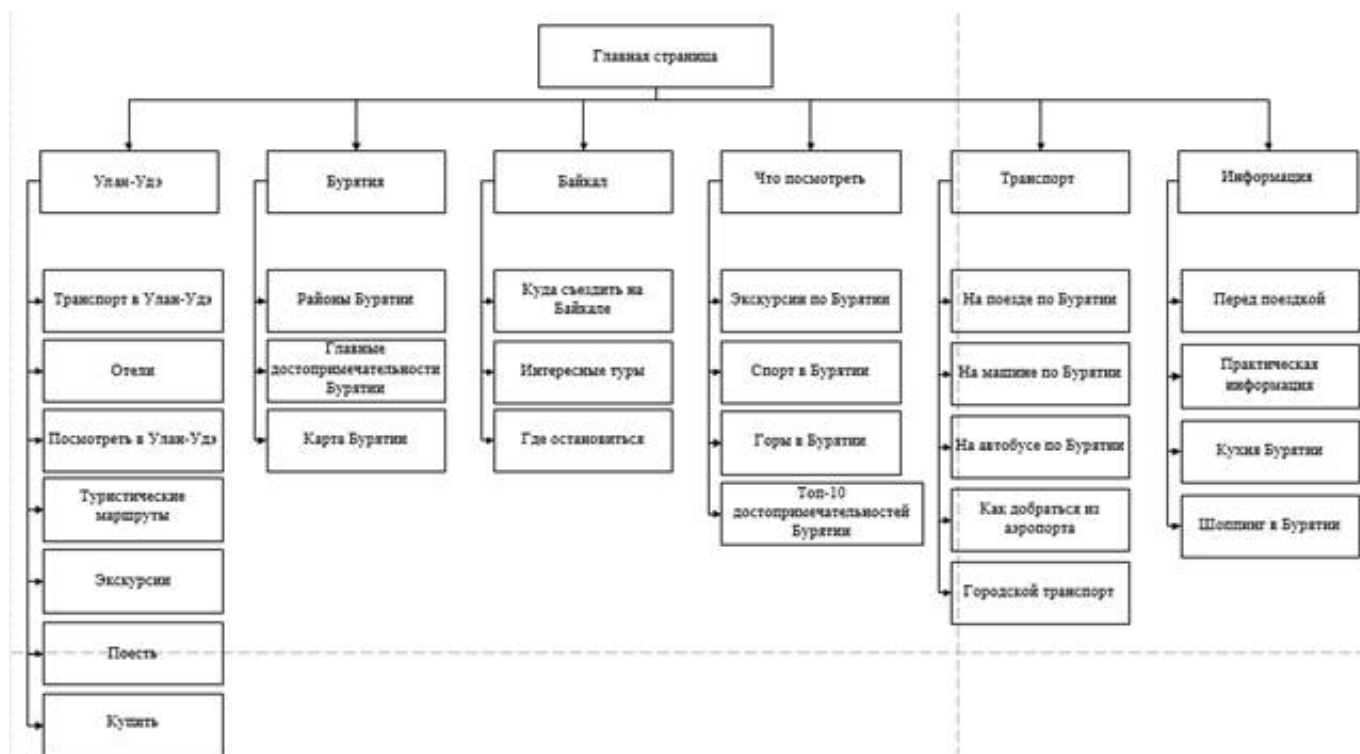
Рисунок 1. Структура сайта
