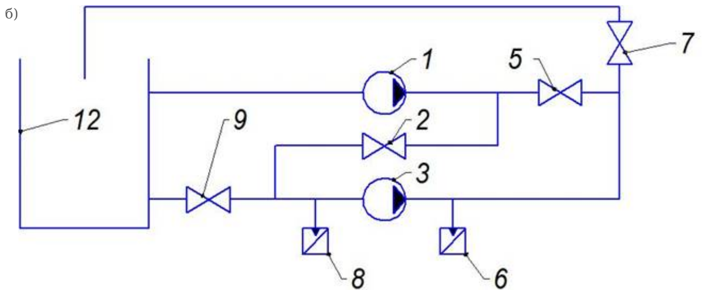
Рисунок 1. Стенд по исследованию рабочих параметров лопастных гидравлических машин: а) 3D модель стенда; б) гидравлическая схема стенда
