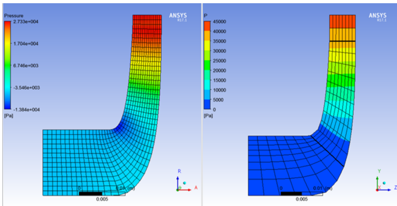
Рисунок 7. Сравнительные диаграммы двух методов расчёта
