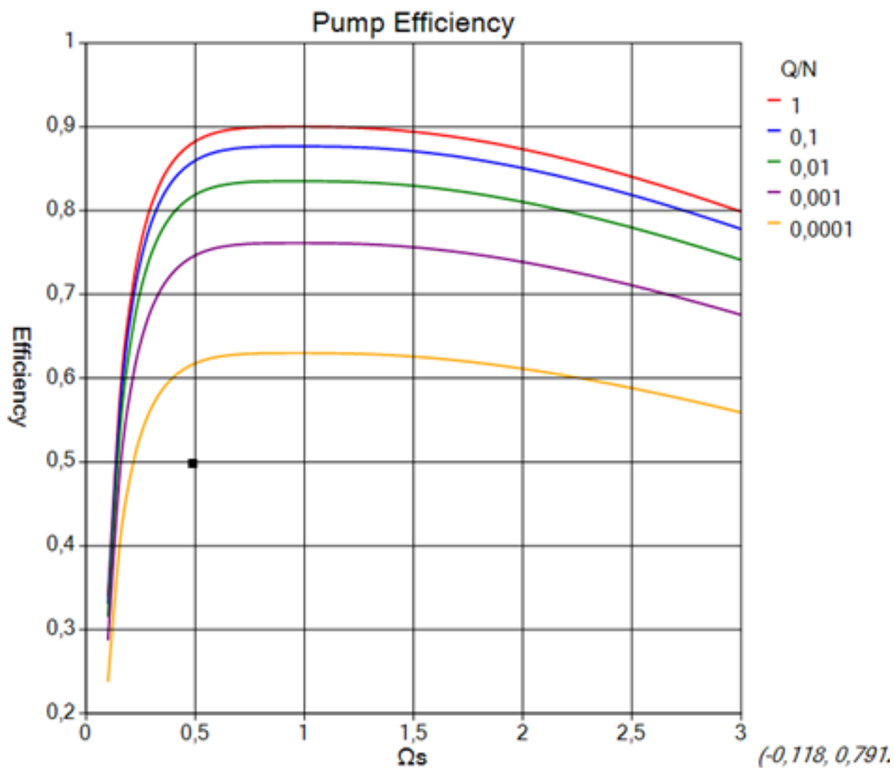
Рисунок 4. График расчётов при одномерном проектировании
