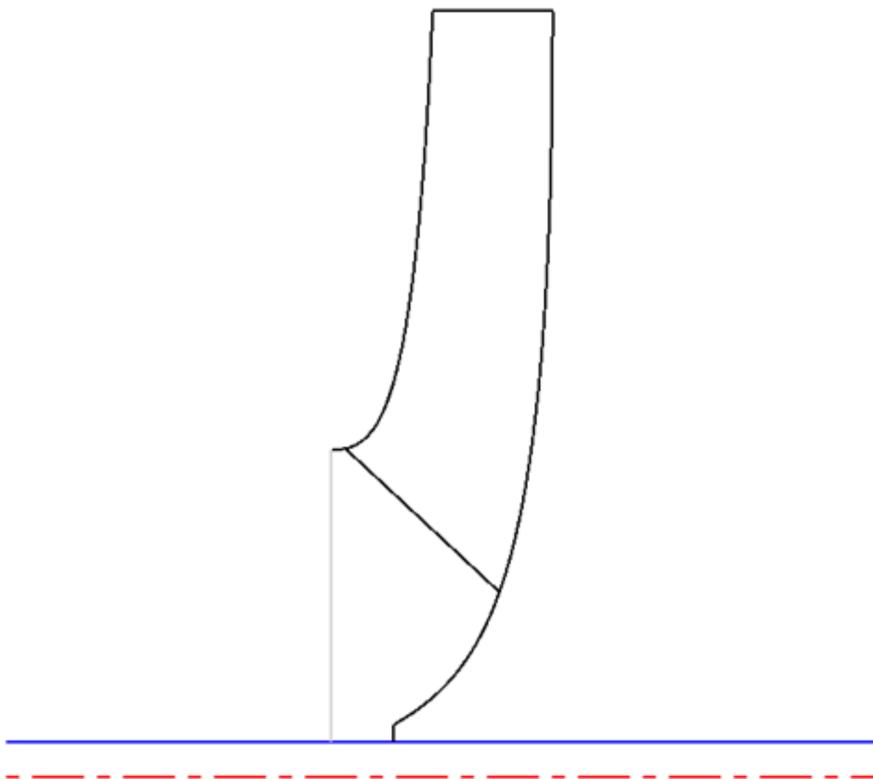
Рисунок 2. Меридианное сечение канала колеса
